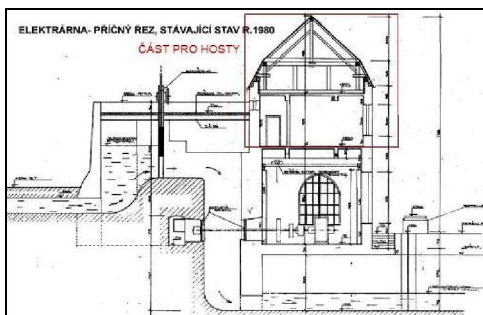
Vlevo část plánu elektrárny (příčný řez) z dokumentace v roce 1980 a fotografie elektrárny v současnosti.
